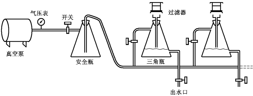
图 8 抽滤系统
